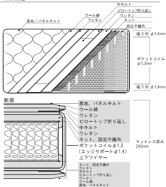
内部構造
